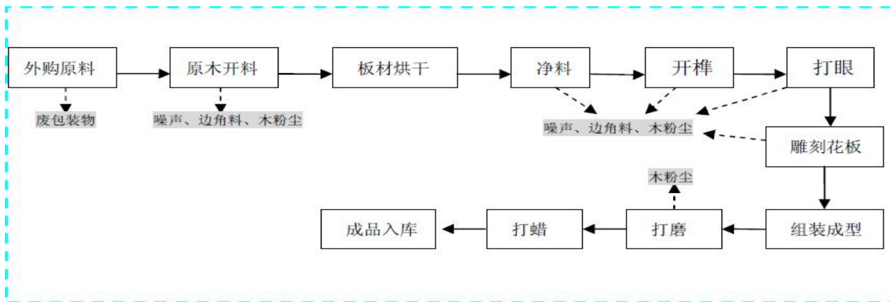
项目生产工艺及产污节点图
