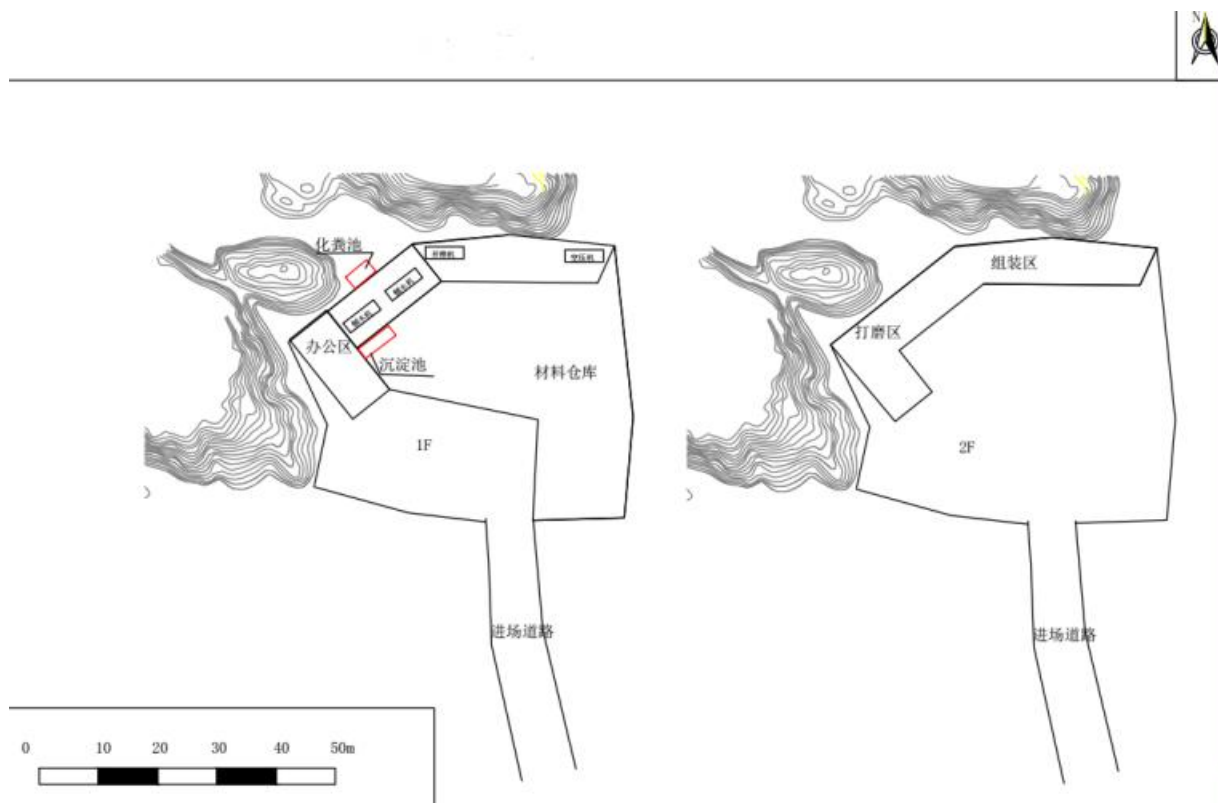
附图 4、项目平面布置图
