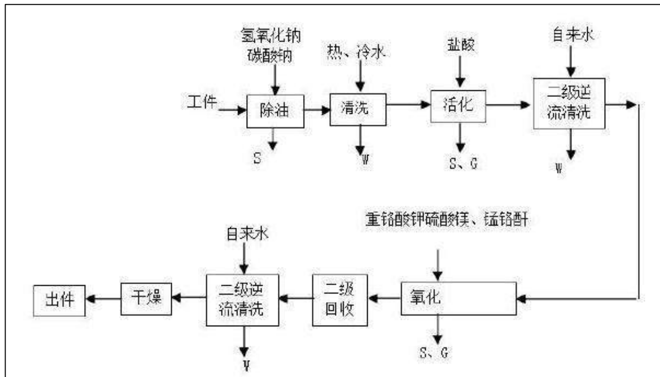
图 1-1 磷化生产工艺简图
